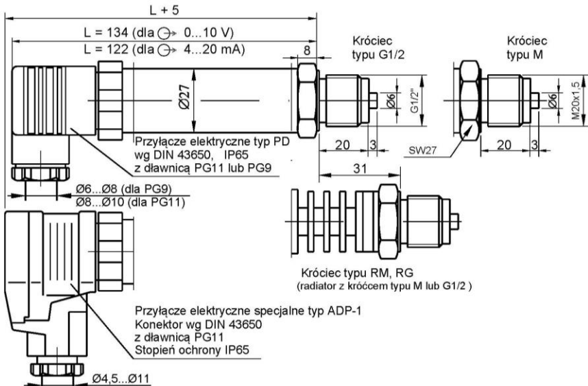
Rys.1. Przetwornik ciśnienia typ AS.
