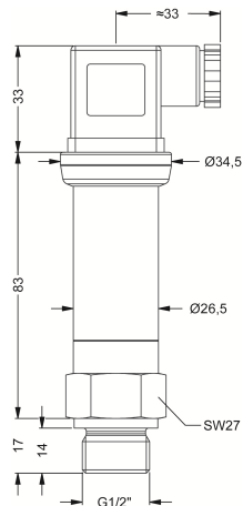
G1/2" DIN 3852
