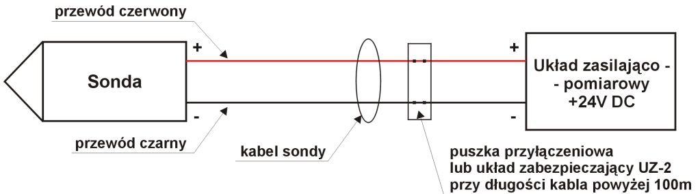
Rys. 5.1. Podłączenie sondy w systemie dwuprzewodowym z sygnałem wyjściowym 4 - 20 mA
