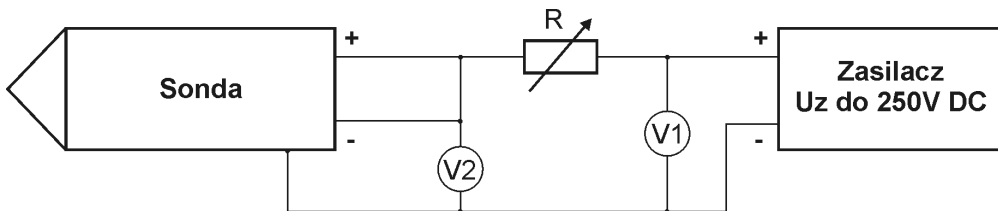
Rys. 7.2. Sprawdzenie iskiernika gazowego
