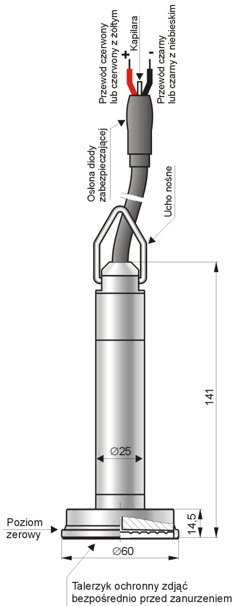
Rys. 1. Wymiary gabarytowe
