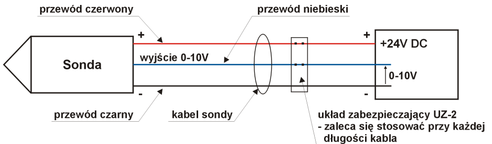
Rys. 5.2. Podłączenie sondy w systemie trzyprzewodowym z sygnałem wyjściowym 0 - 10 V
